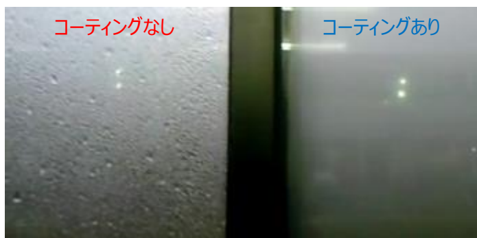
IRUVカットコート未塗布・塗布の結露(2時間)
